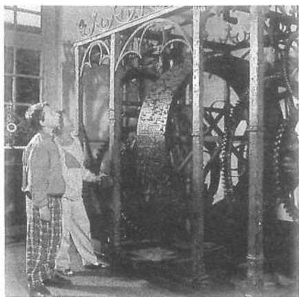
Toren uurwerk / Tower clock 1542 Heynrick Vabrie, Breda
